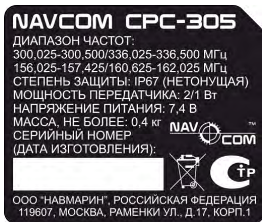
Рисунок 1 – Маркировка радиостанции
