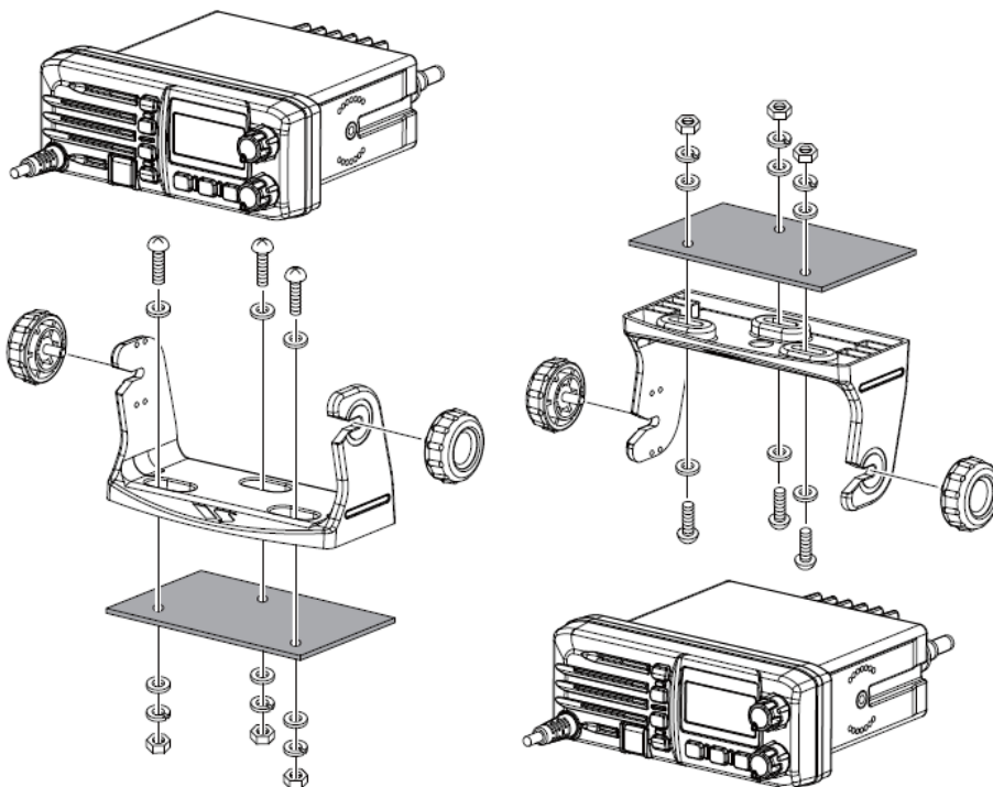
Настольная установка
